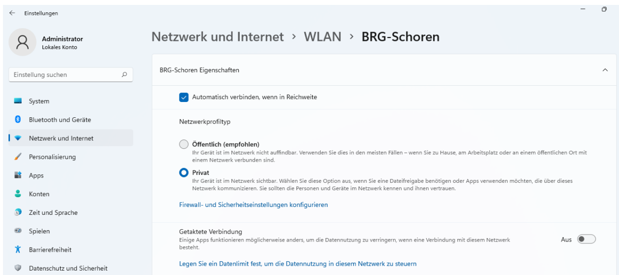
Abbildung 6: Netzwerkprofiltyp ändern
