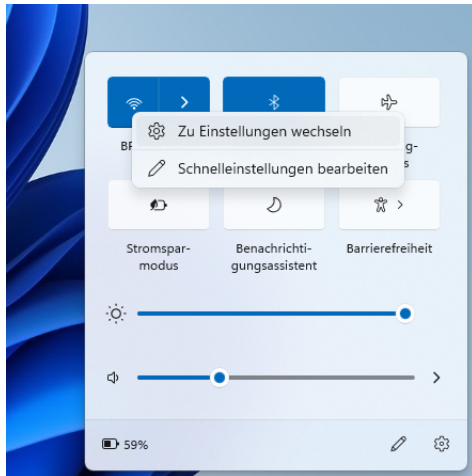
Abbildung 5: WLAN Einstellungen
