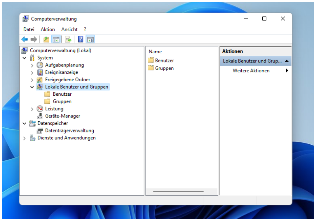
Abbildung 3: Benutzerkonten anlegen
